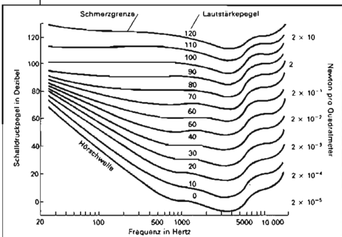
Die Kurven gleicher Lautheit, auch Fletcher-Munson-Kurven genannt.
